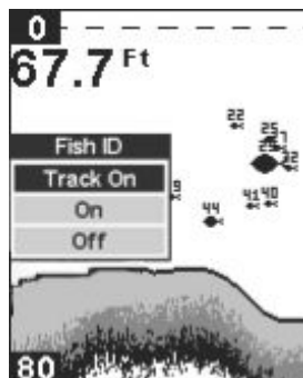
Меню FISH ID и символ рыбы при включенной функции FISH TRACK. Рыба на глубине 44 фута.
